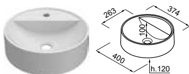
PURO T ROUND pultra ültethető mosdó
