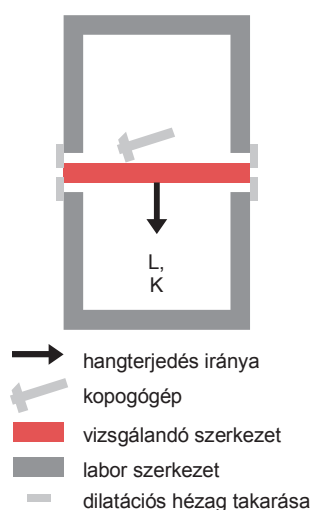
A3 A kerülőút nélküli, laboratóriumi szabványos lépéshangnyomásszint értelmezése
