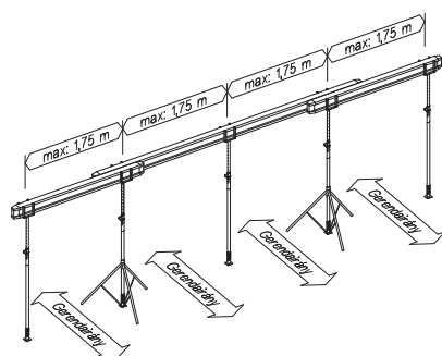
4 Gerendák alátámasztása és túlemelése csőállvánnyal
