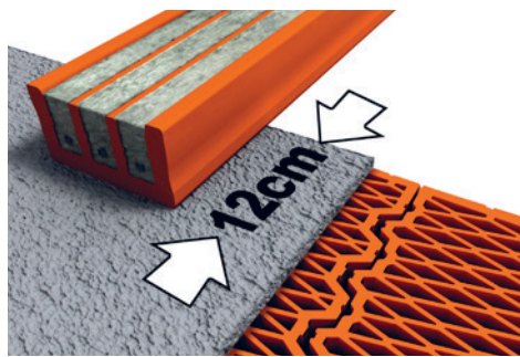
6 A gerendák elhelyezése
