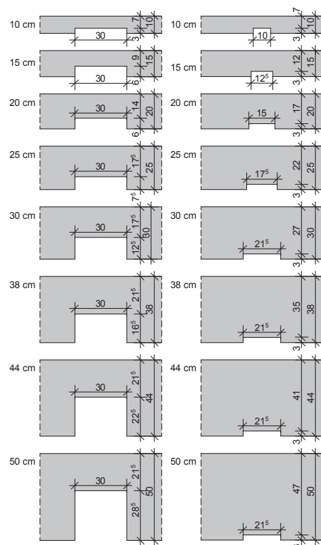
A falazat építése során készített falhornyok és falbeugrások
