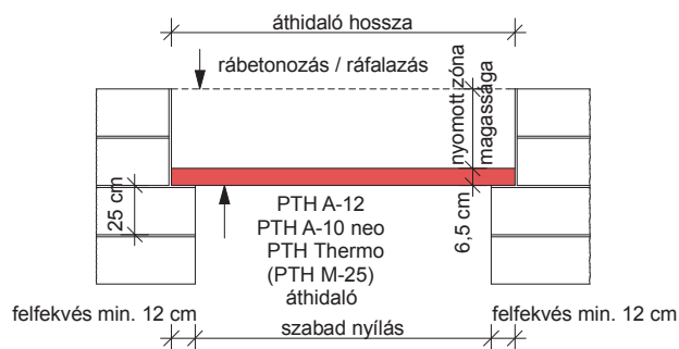
kompozit áthidaló szerkezet
