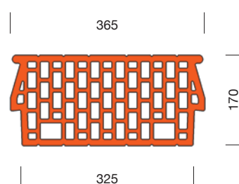
Porotherm 45/17 béléstest
