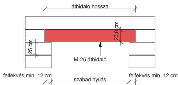
egyszerű áthidaló szerkezet
