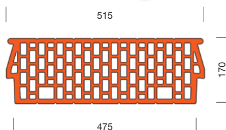
Porotherm 60/17 béléstest
