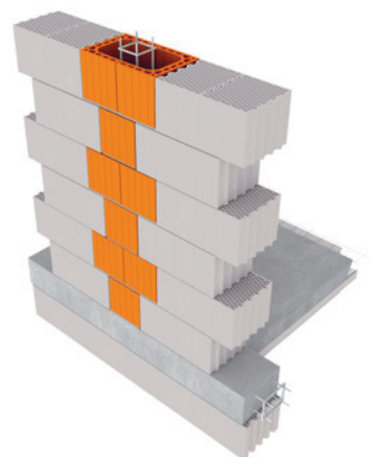
Függőleges zsaluzatként, téglakötésben
