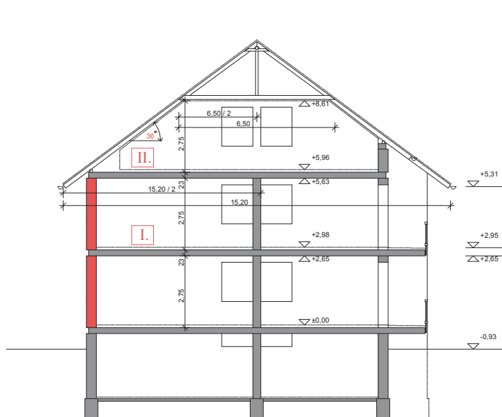
Sematicus metszet
