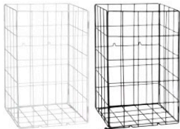
Szemetes kosár Wire basket, steel 350×550×265 mm
