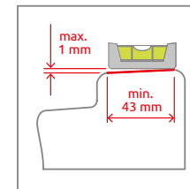
Zuhanytálcára szerelés esetén a zuhanytálca szélének szélessége min. 43 mm és a dőlésszögének max. 1 mm lehet.
