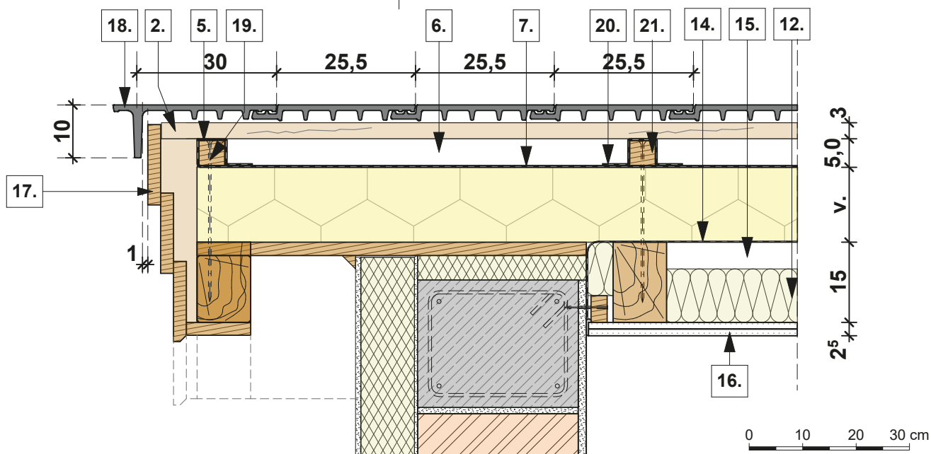
Orom részletrajz
