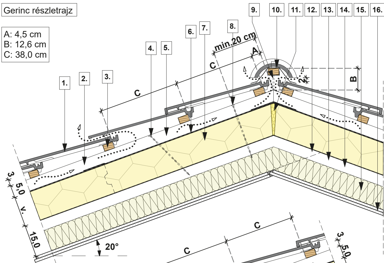
Eresz részletrajz
