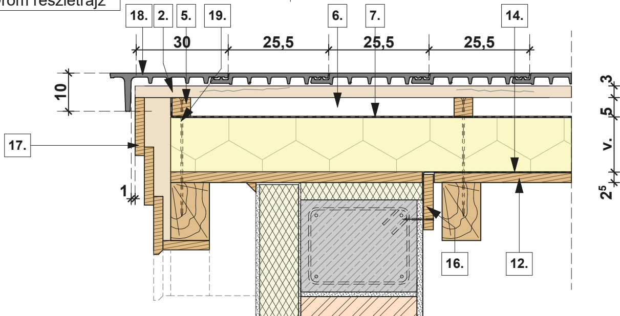
Orom részletrajz
