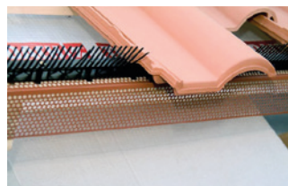
eresz szellőzőfésű
