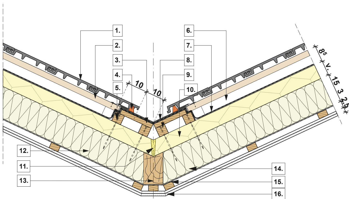
Orom részletrajz
