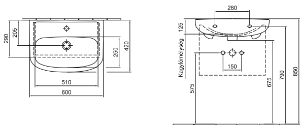
Beépíthető mosdó 6006 33 xx
