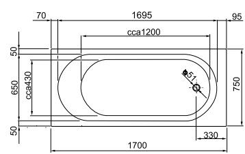
CASSANDRA 170 x 75 cm klasszikus fürdőkád UBA170CAS2P-01
