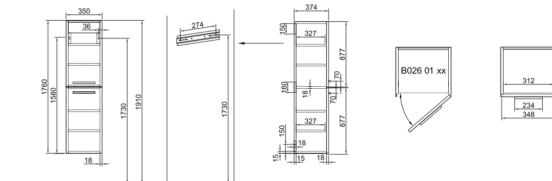
Magasszekrény B026 01 xx
