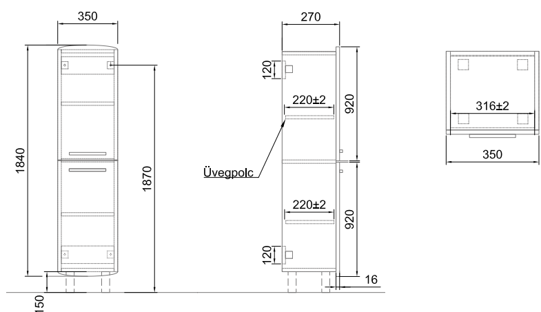
Tükrösszekrény világtás nélkül A498 60 xx
