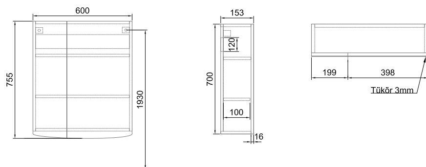
Tükör világtás nélkül A499 60 xx
