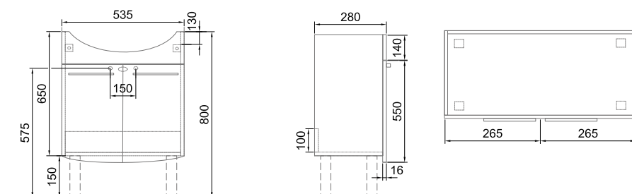
Mosdószekrény A897 xx xx
