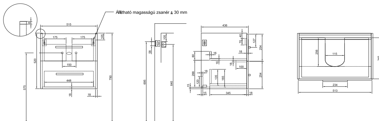
Magasszekrény B026 00 xx
