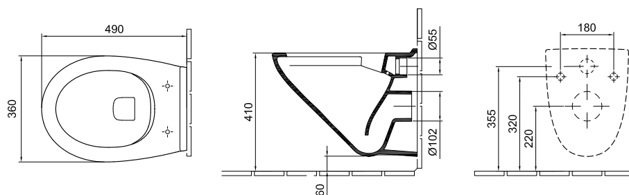
Méylöblítésű falí-WC 7048 R0 xx
