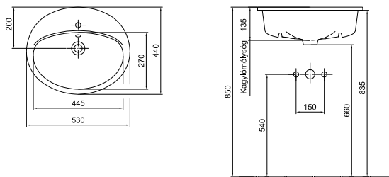
Kézmosó 7332 5X xx
