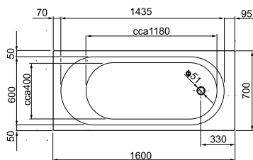
CASSANDRA 160 x 70 cm klasszikus fürdőkád UBA160CAS2P-01
