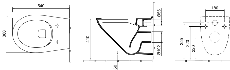
Méylöblítésű falí-WC 7048 R0 xx
