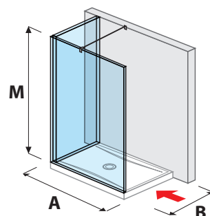
ÜVEGFA PURE „L” 120, 130, 140 × 80 cm | 120, 130, 140 × 90 cm
