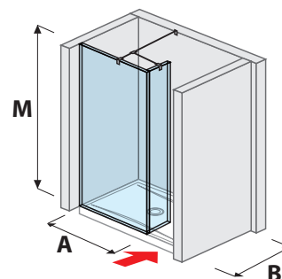
üvegfal PURE rövid üvegfallal 70, 80 cm
